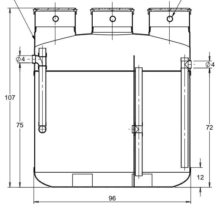
SECTION A-A SCALE 1 : 35
